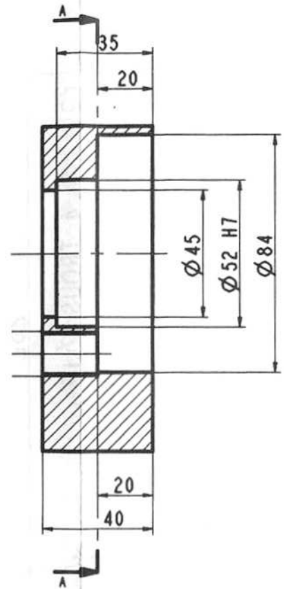
COUPE B-B
