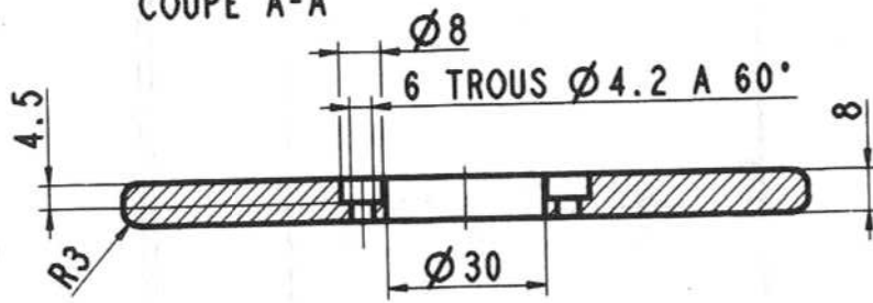
COUPE A-A
