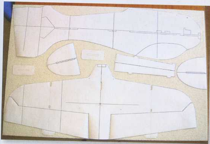
Les gabarits en papier pour la découpe.
