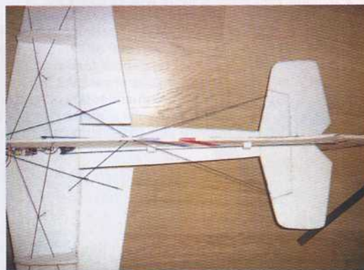
Le haubanage complet de la cellule.
