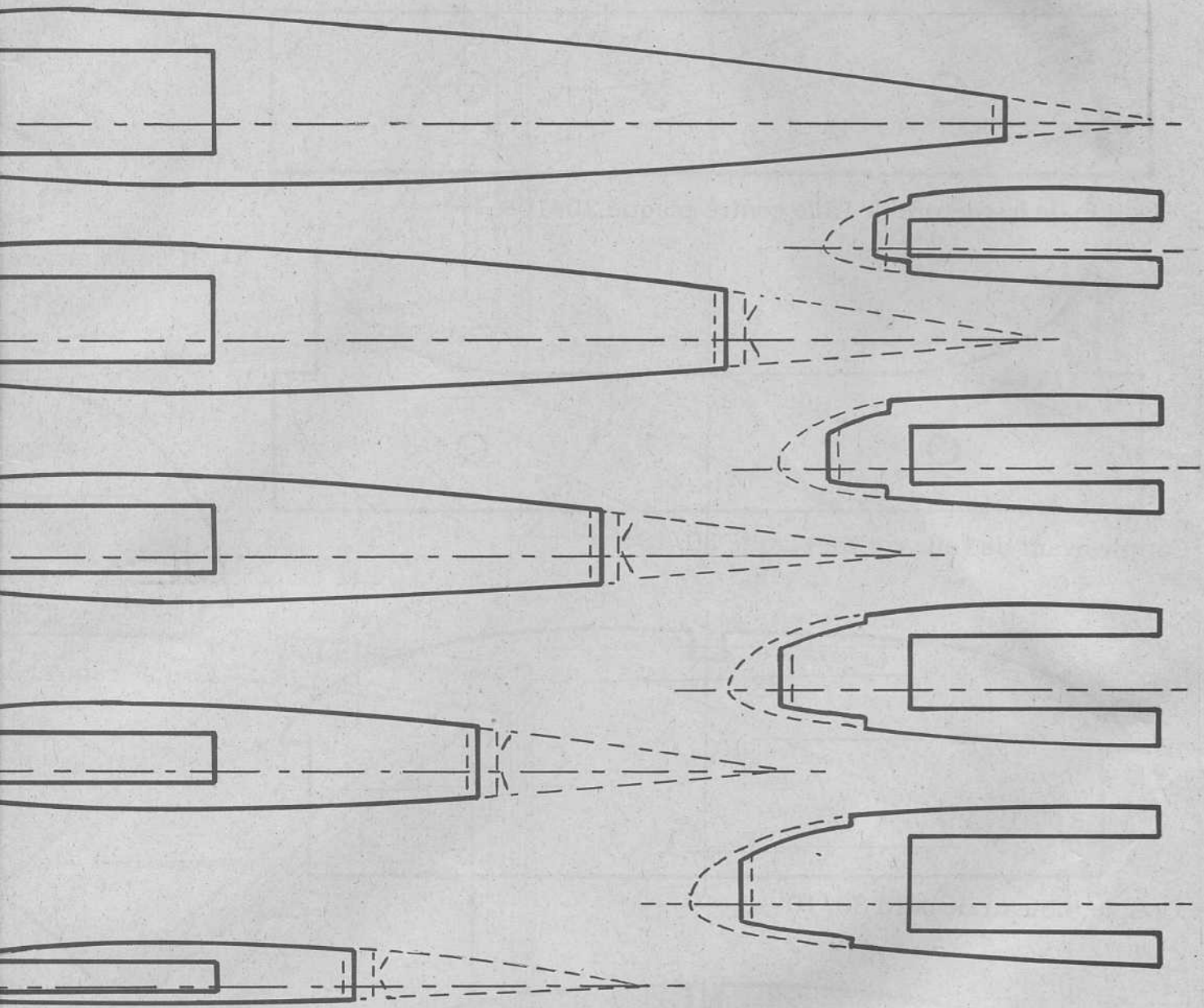
Nervures et demi-nervures 20/10
