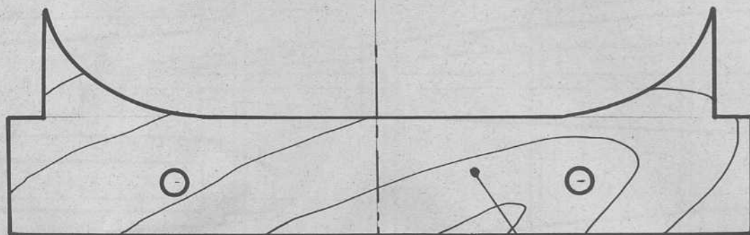
Couple avant de l'aile contre-plaqué 30/10
