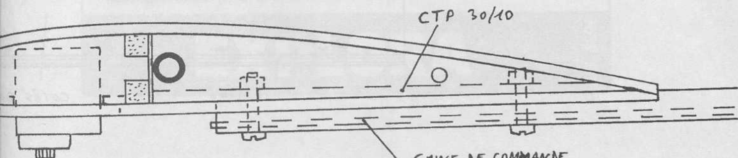
COUPE D-D
