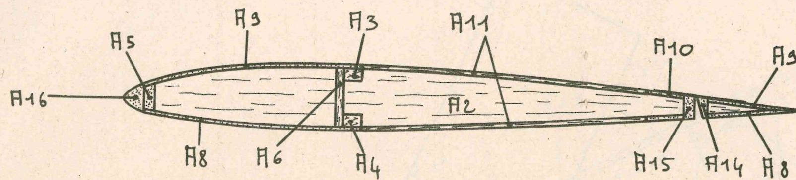
Coupe H-H.
