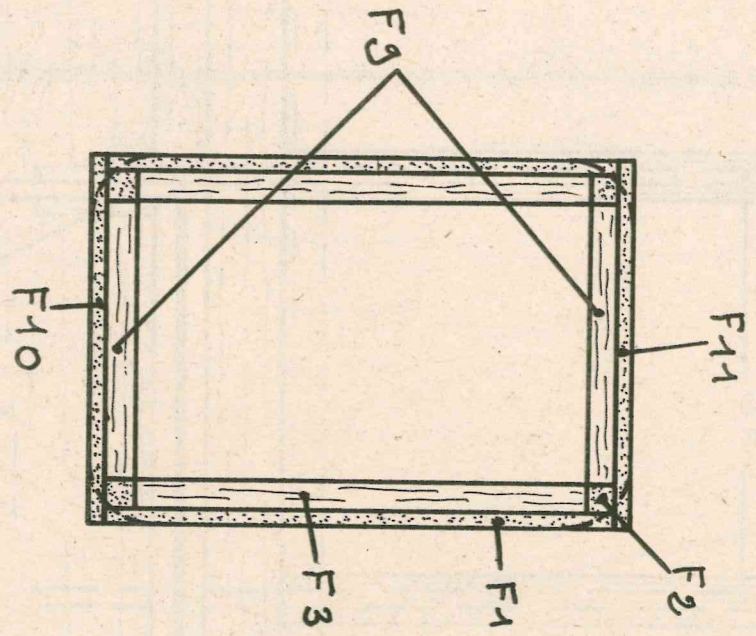
Coupe F-F.
